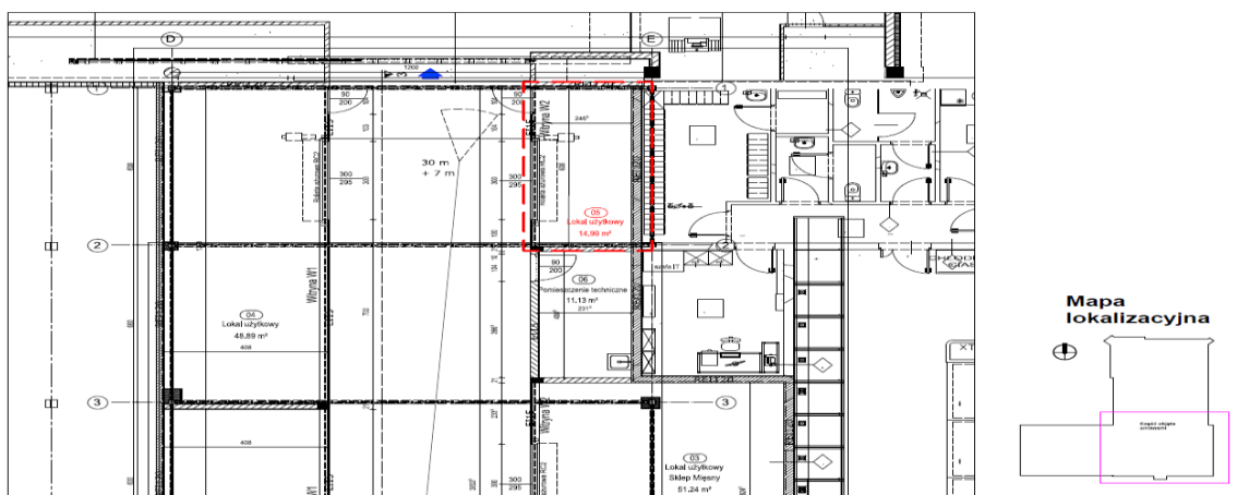
Rzut przyziemia nr 1
